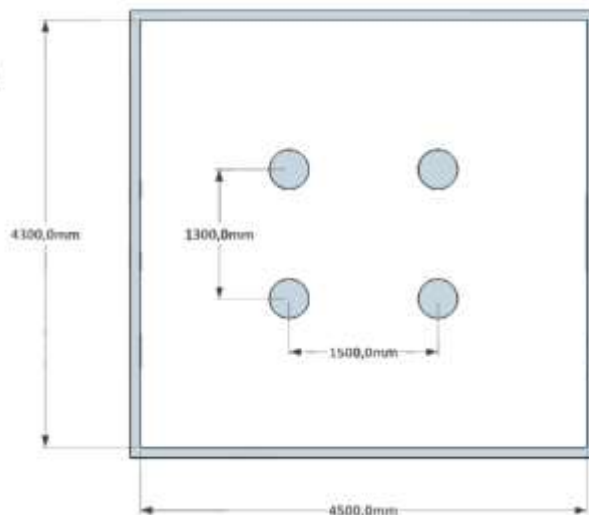
HB-1002 Babaház OKO-val Betonozási pontok
